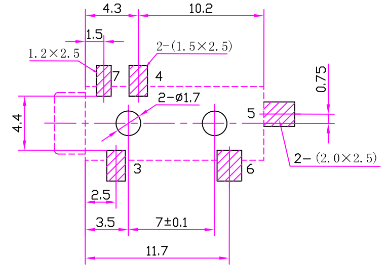
线路版安装位置图
